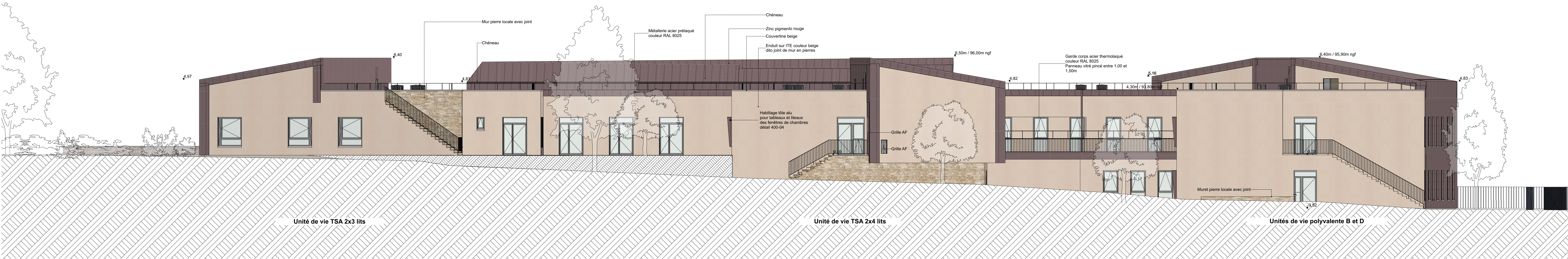
Façade Sud
